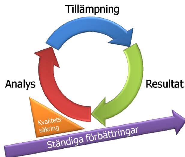
Figur 1-1: Systematiskt kvalitetsarbete
