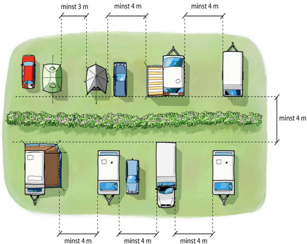
Rekommenderade säkerhetsavstånd.
